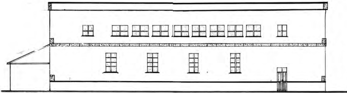
FACHADA SUR. 20 metros
